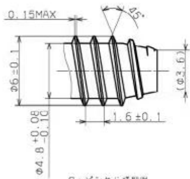
タッピンねじ詳細図 DETAIL OF TAPPING SCREW
