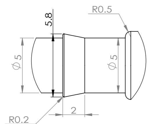
局部视图 B 比例 5:1
